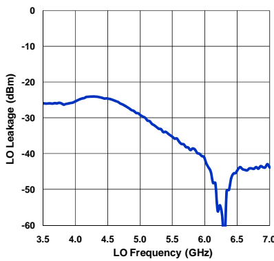
LO Leakage
