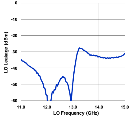
LO Leakage
