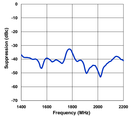
Sideband Suppression
