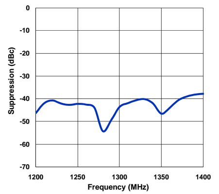
Sideband Suppression
